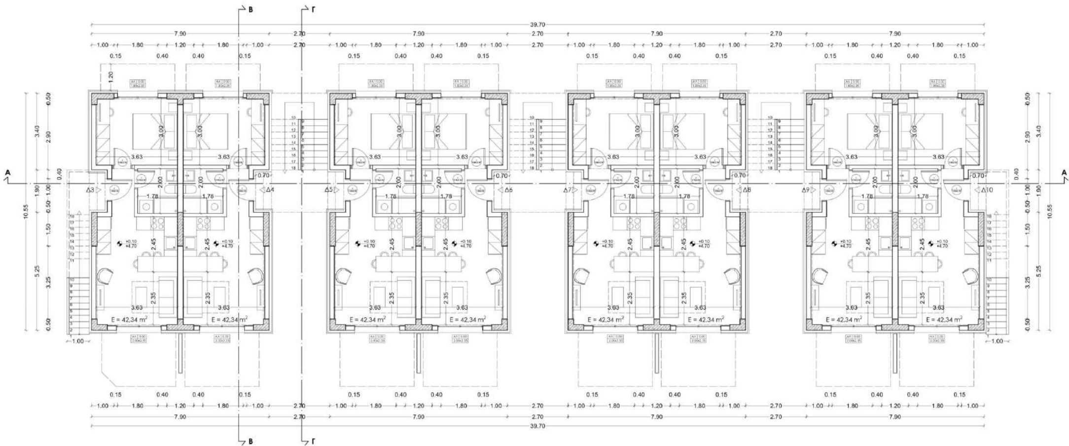
ΚΑΤΟΨΗ ΙΣΟΓΕΙΟΥ
