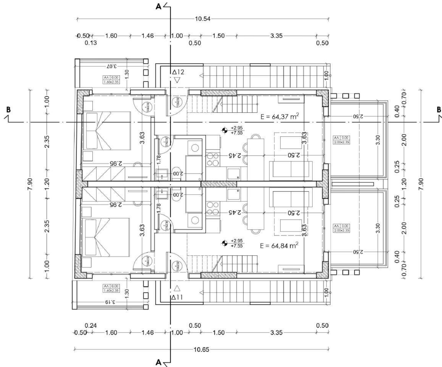
ΚΑΤΟΨΗ ΟΡΟΦΟΥ
