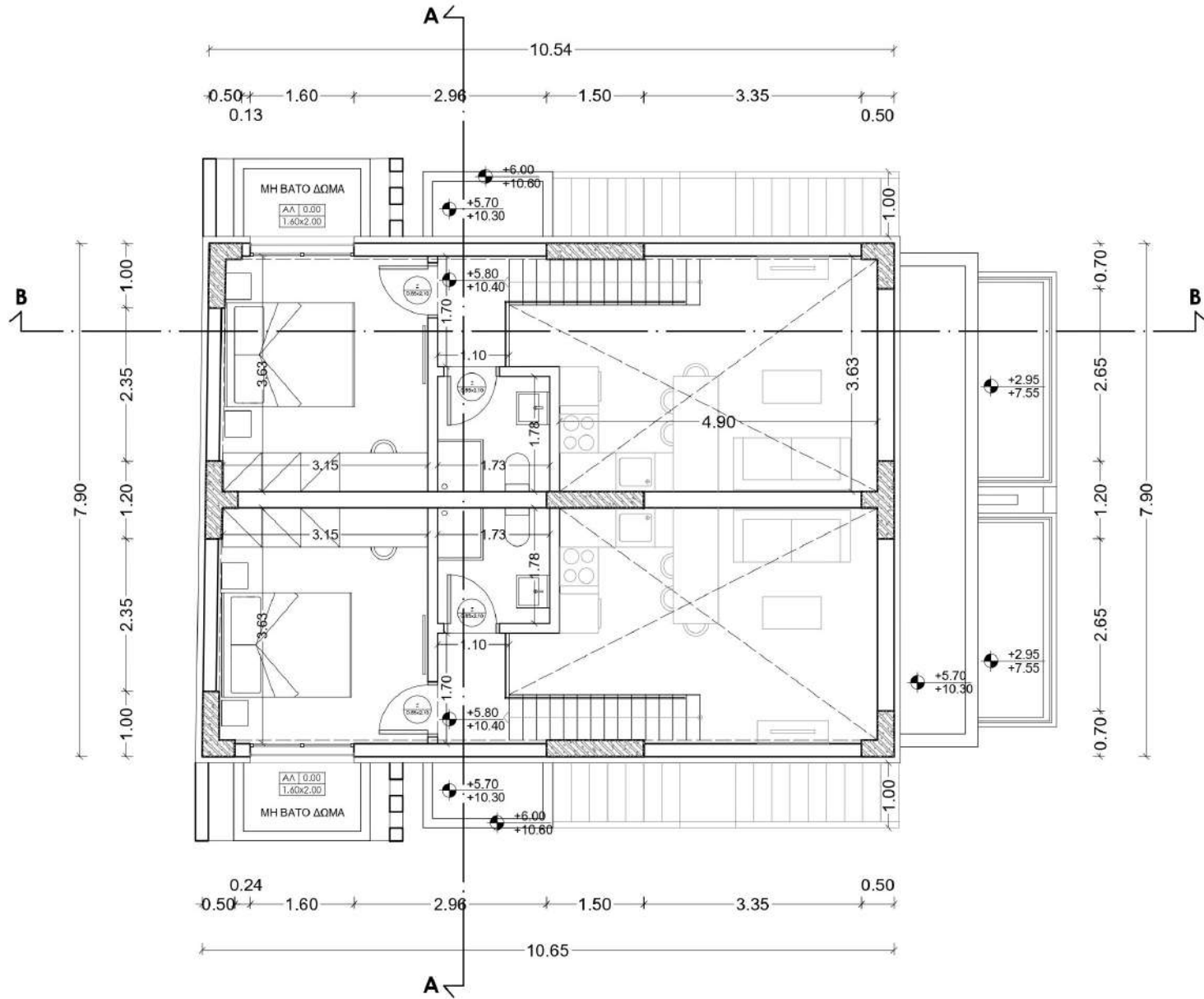
ΚΑΤΟΨΗ ΣΟΦΙΤΑΣ
