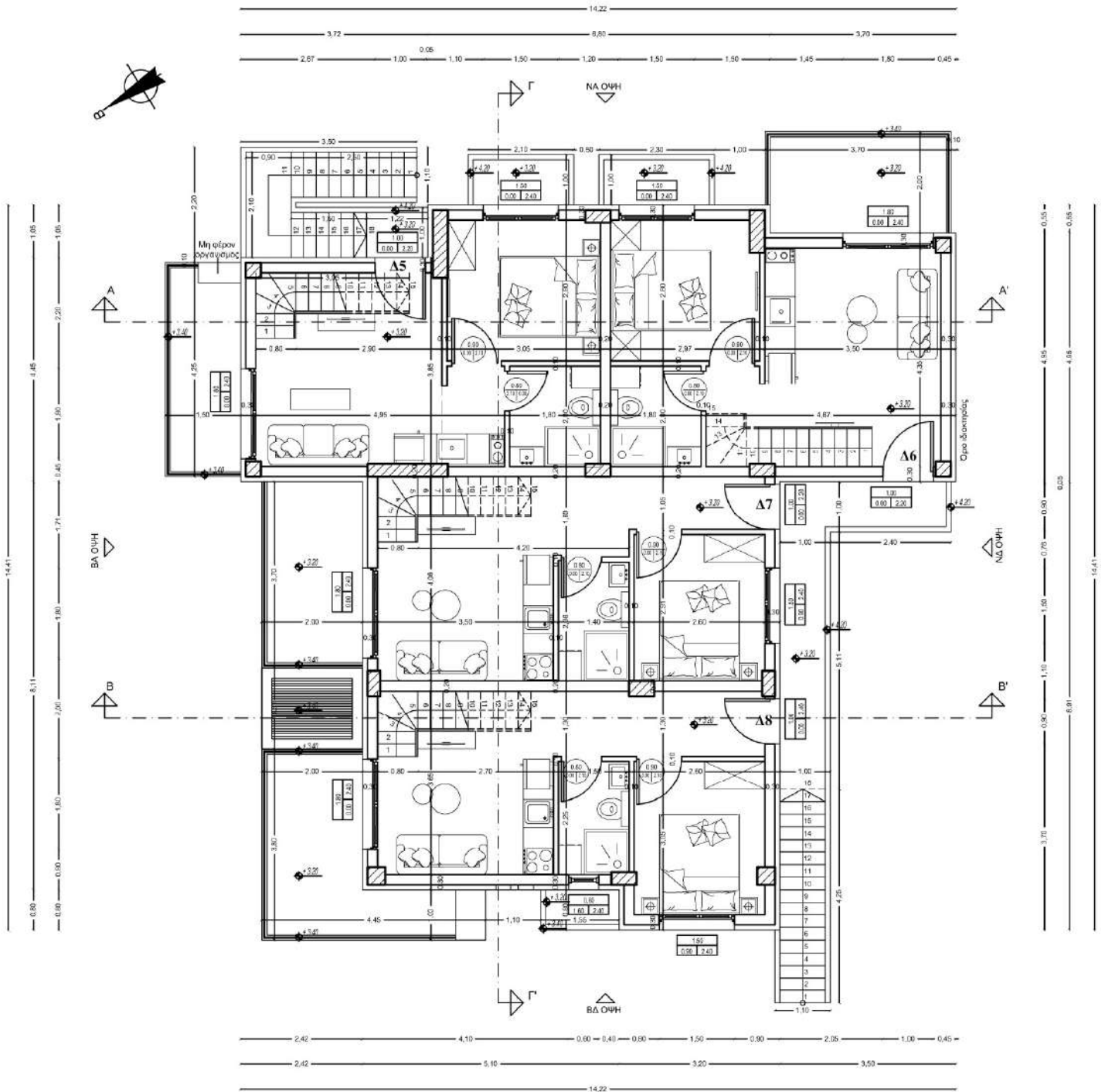
ΚΑΤΩΦΗ ΟΡΟΦΟΥ
