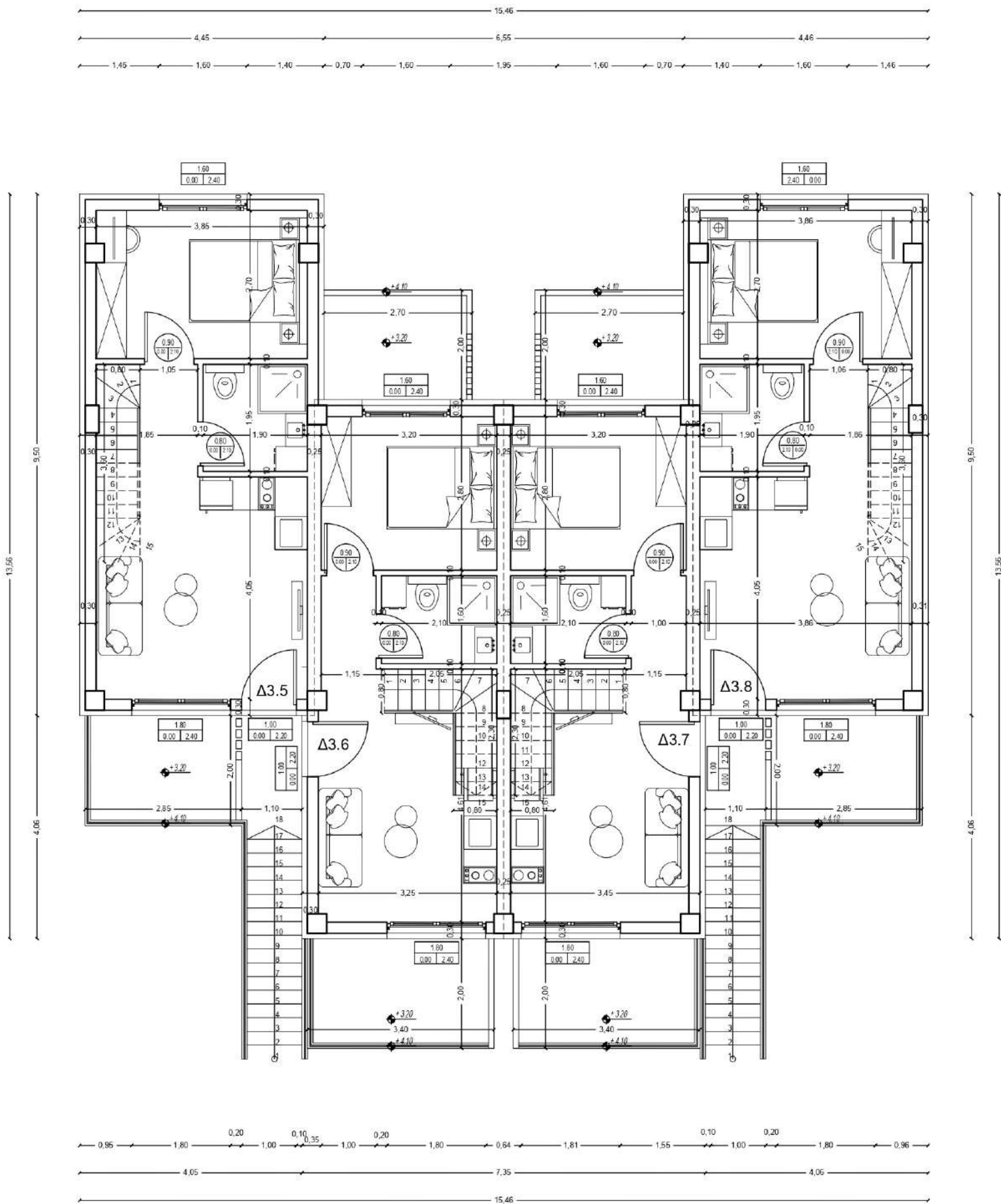
ΚΑΤΩΦΗ ΟΡΟΦΟΥ
