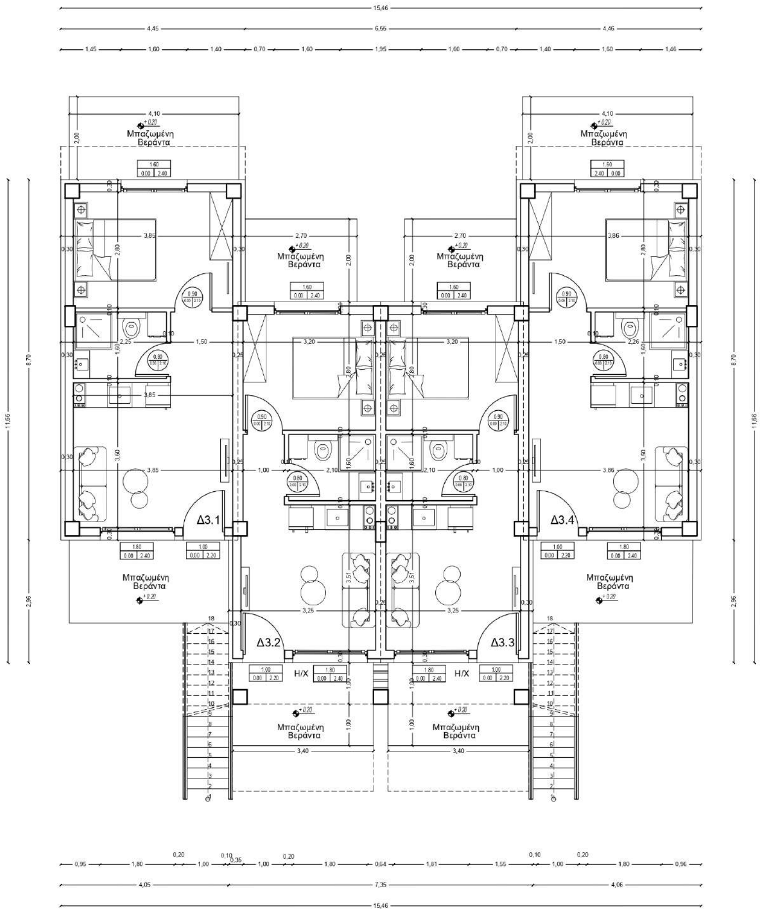
ΚΑΤΟΠΗ ΙΣΟΓΕΙΟΥ
