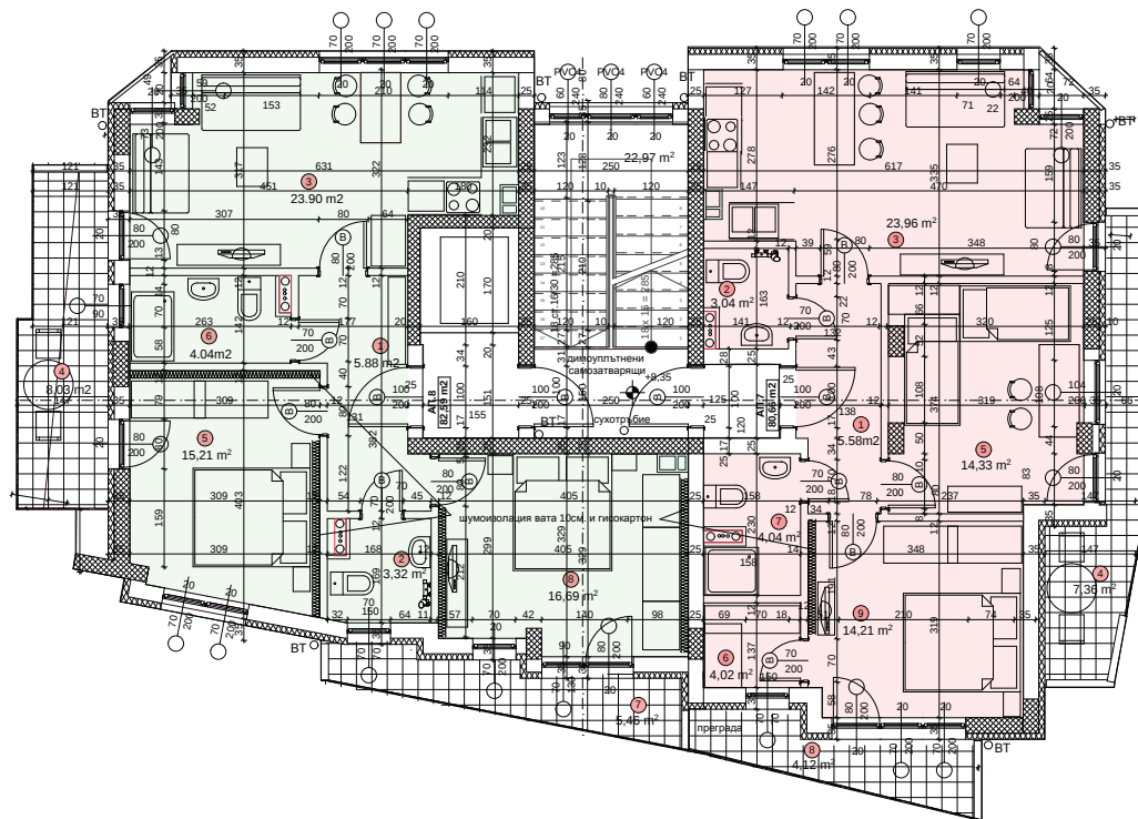
Апартамент 8 / 101,38 кв.м.
