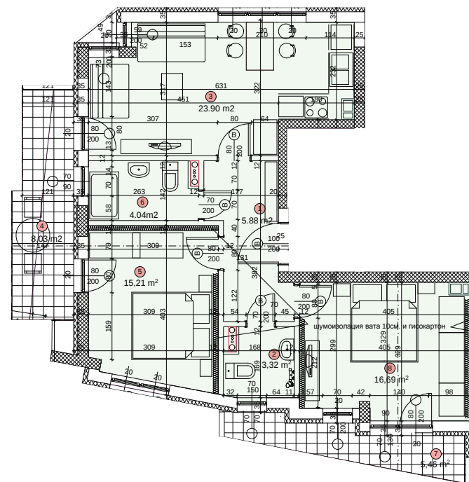
Апартамент 8 / 101,38 кв.м.
